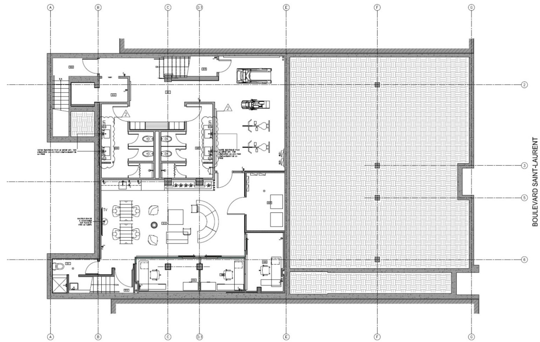
SOUS-SOL | BASEMENT
